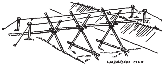
LØBEBRØ MED UNDERLAG AF FIRE RAFTER
