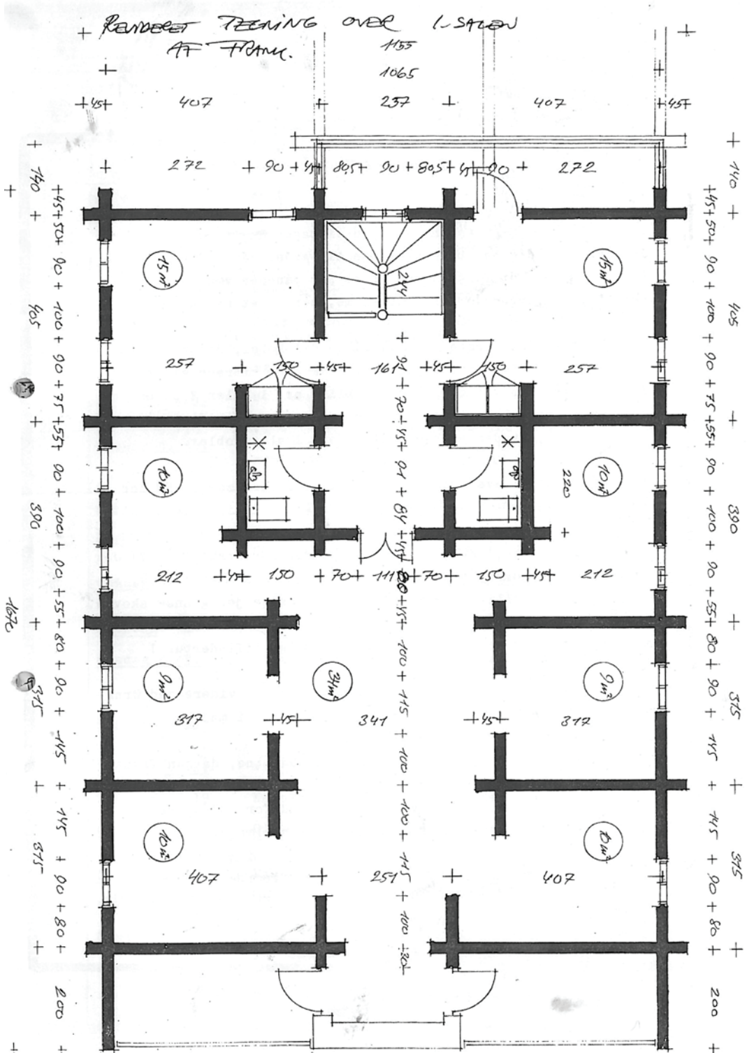
Revideret tegning af 1. sal. Hytten er tegnet af Frank Juncker
