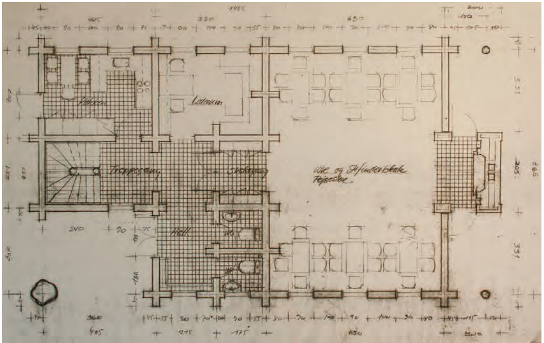
Plantegning af stueetagen til den endelige hytte
